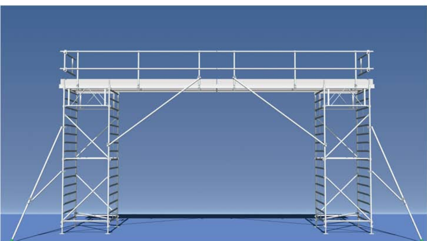
Één of twee werkbrug(gen) naast elkaar op Layher renovatietorens. Een ideale combinatie voor werkzaamheden aan daken en gevels.
